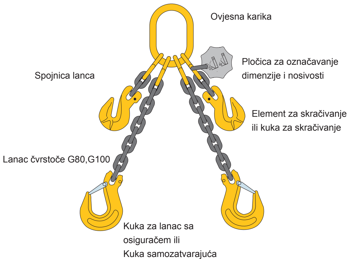
Komponente lančane priveznice - 6;7;8;10;13;16;18;20;22;26mm
