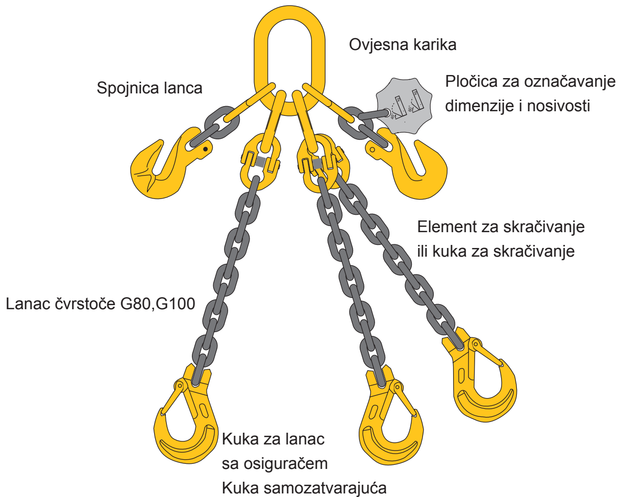
Komponente lančane priveznice trokrake 6;7;8;10;13;16;18;20;22,26mm
